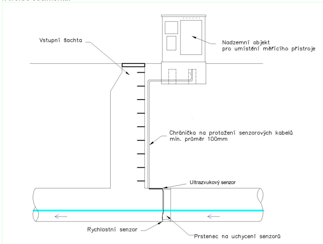
Schéma měrného objektu na stoce
