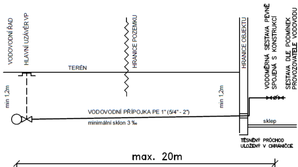
PODÉLNÉ SCHÉMA
