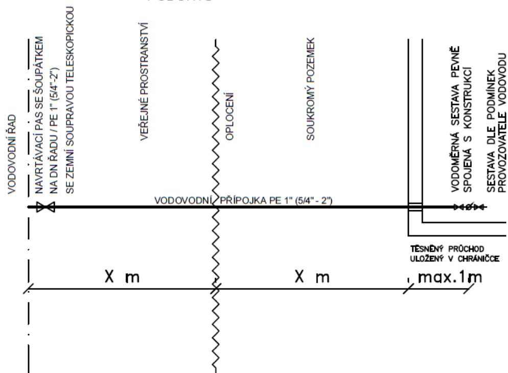
PŮDORYS
