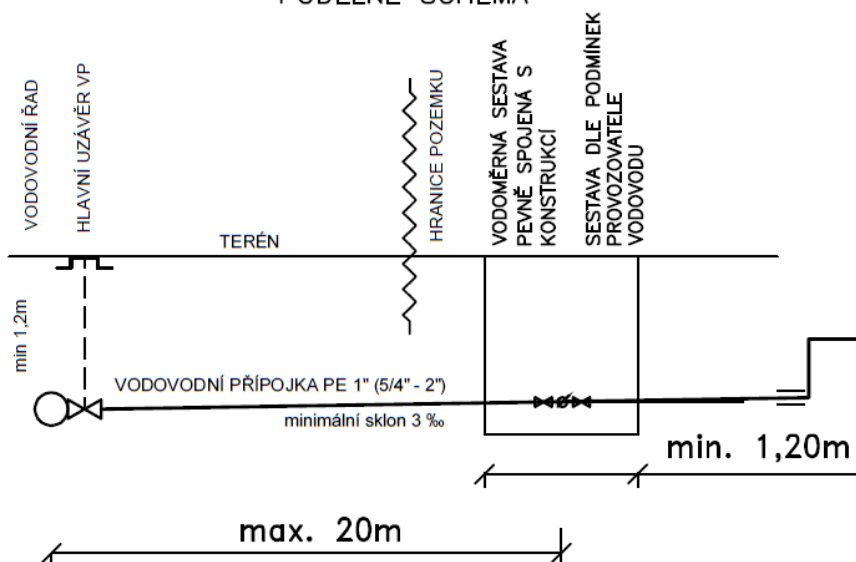
PODÉLNÉ SCHÉMA
