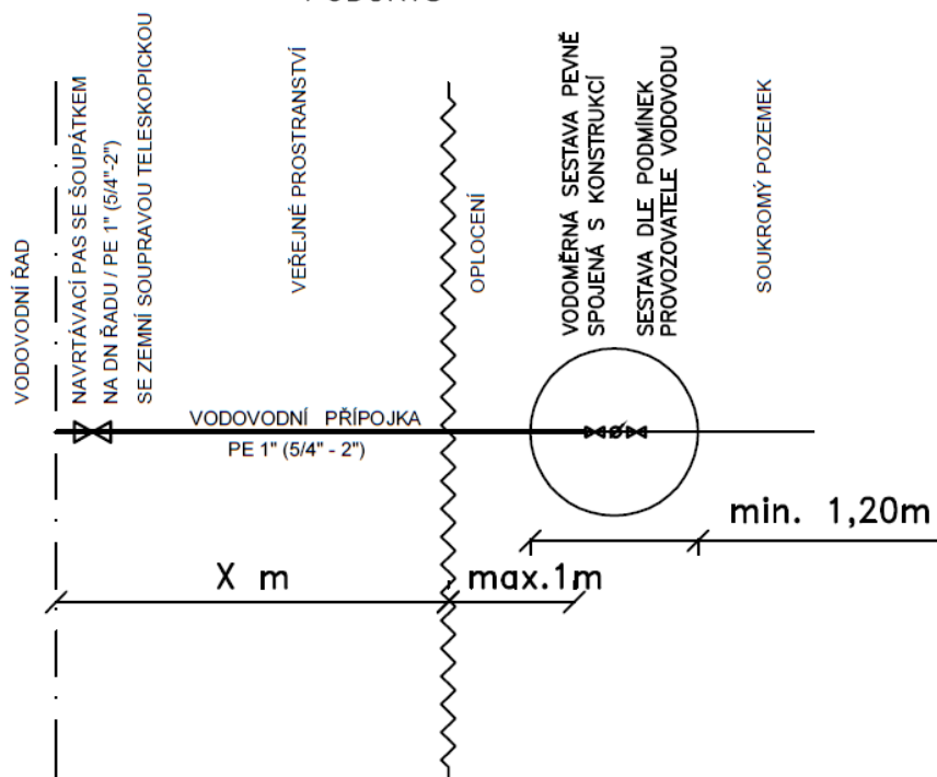
PŮDORYS
