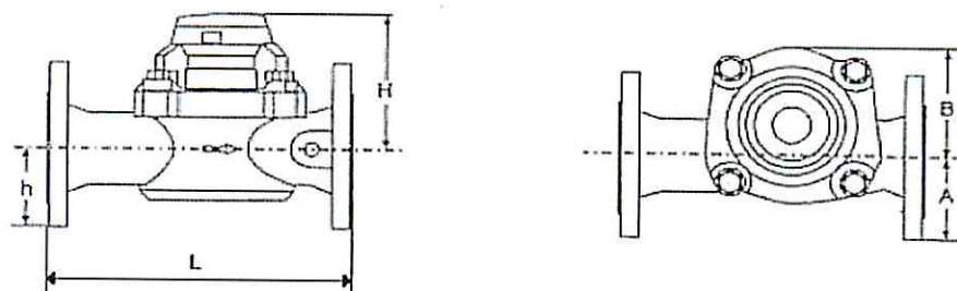
V8 – Vzorová vodoměrná šachta „plastová“
